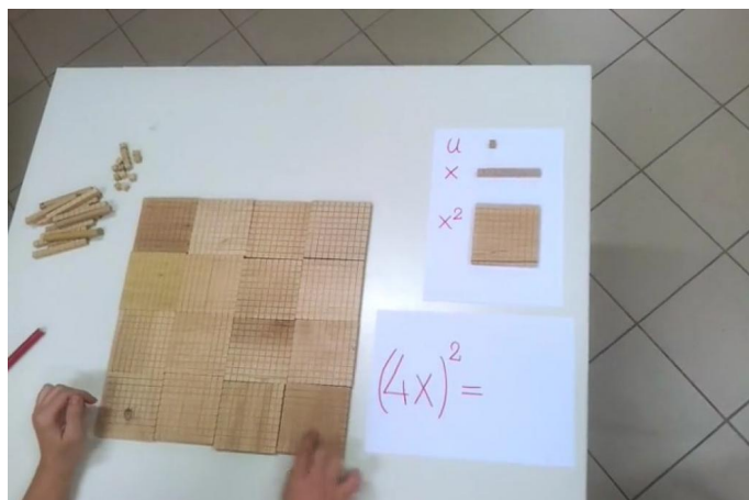
Calcolo quadrato monomio
